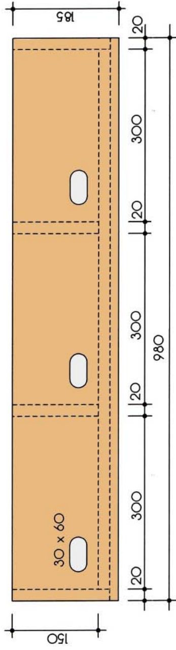
Ansicht Frontplatte
